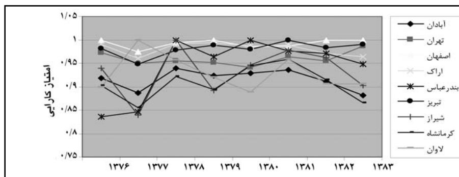
نمودار ۱۰ منحنی کارایی پالایشگاه‌های نفت کشور در سال‌های ۸۳-۷۶
