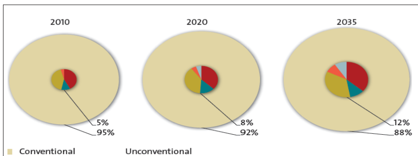
شکل ۶ | سهم تولید نفت نامتعارف از کل تولید نفت خام جهان در سال های ۲۰۱۰، ۲۰۲۰، ۲۰۳۵ و [۱۴]
